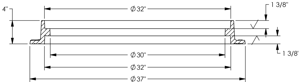
SECTION A-A
