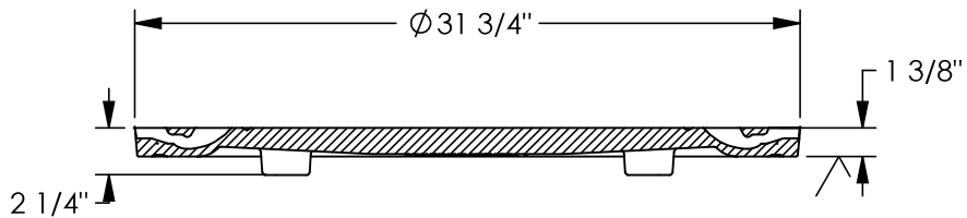
SECTION A-A
