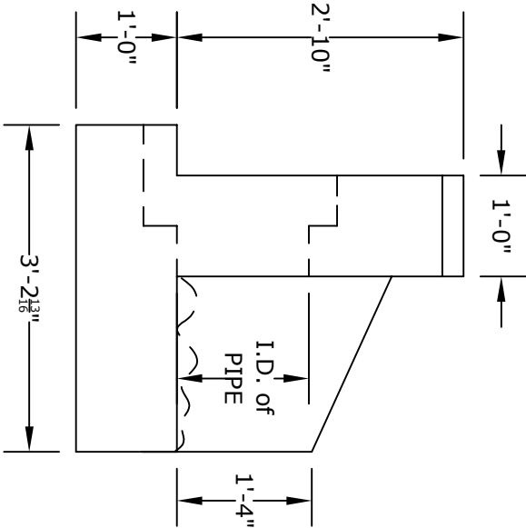
ELEVATION B
